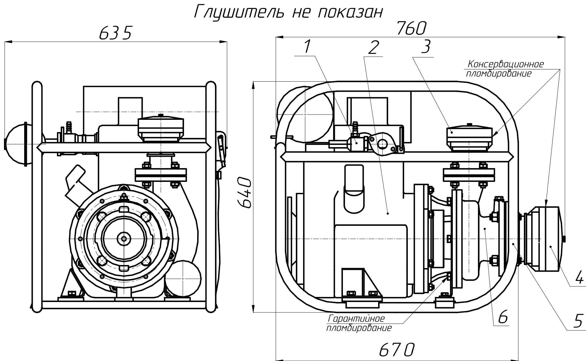
Рисунок 1 - Общий вид мотопомпы типа МД. 1 - Газоструйный аппарат; 2 - Дизельный двигатель; 3 - головка напорная ГЦ- 50; 4 - Головка всасывающая ГМВ-80; 5 - Рама; 6 - Насосная часть.
